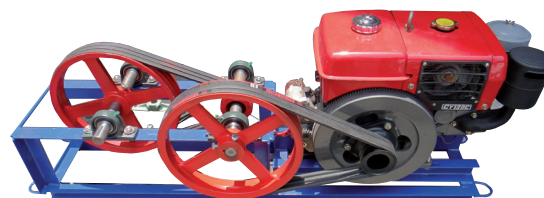
Reductor reforzado..
