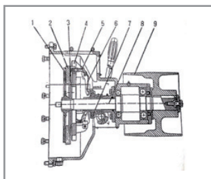
Embrague
