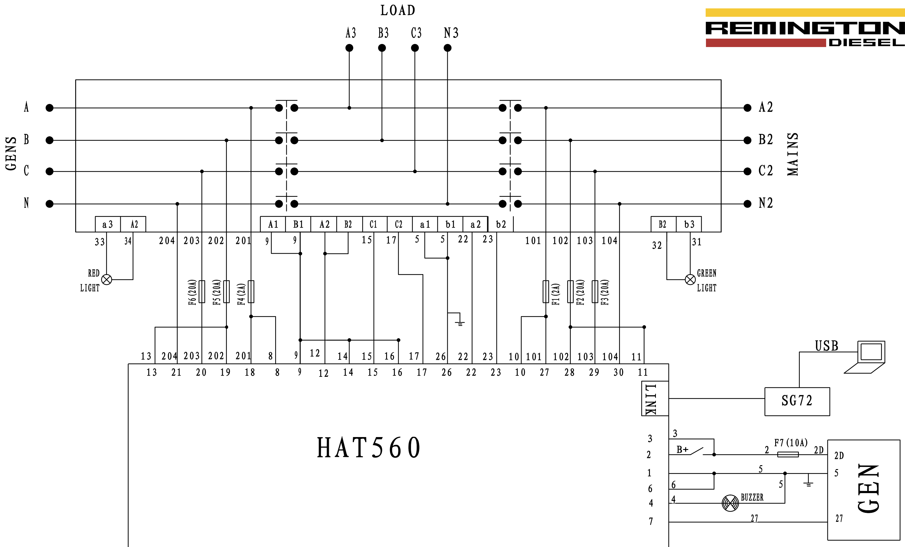
ATS Wiring Diagram HAT560 Model: 250GFS
