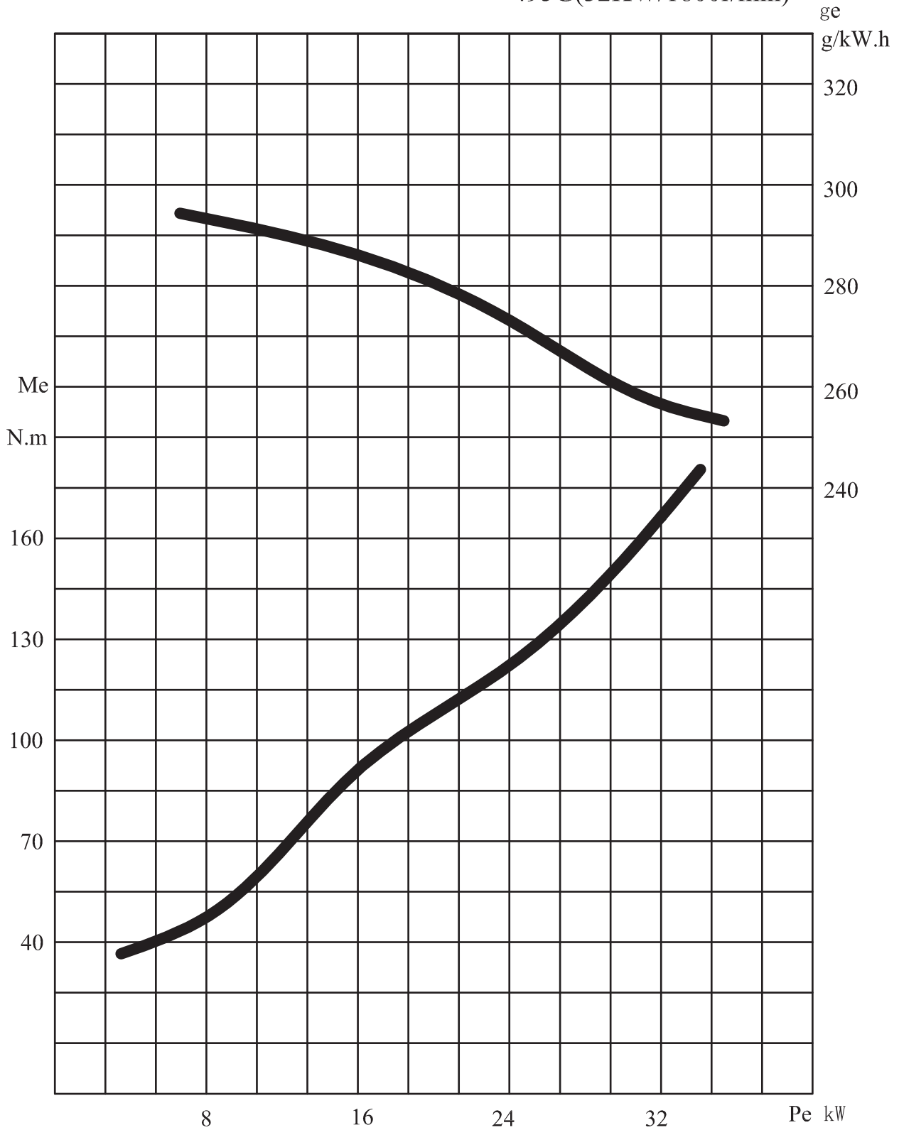
495G(32KW/1800r/min)
