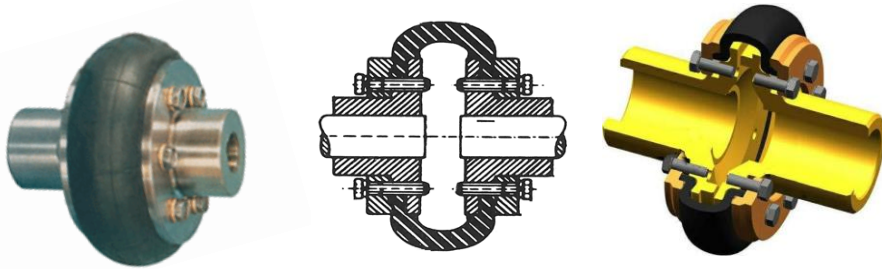
Matrimonios / Acoples industriales tipo Llanta
