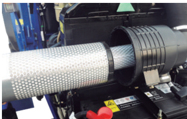
Filtro de aire Donaldson seco doble con prefiltro incorporado.
